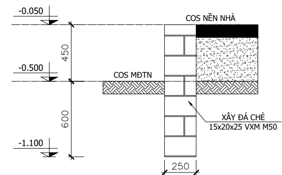
MÓNG ĐÁ CHÈ MD TL: 1/25
