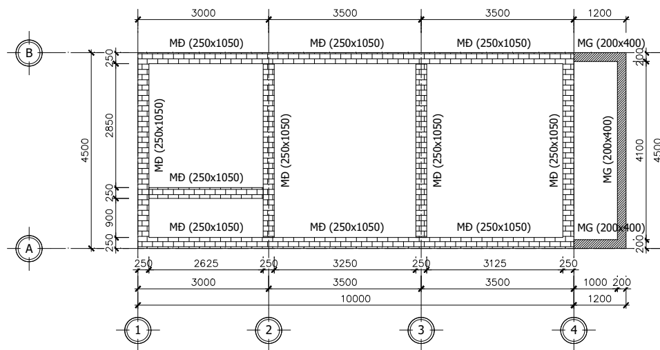
MẶT BẰNG MÓNG ĐÁ CHÈ TL: 1/100
