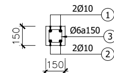
GIẺNG TƯỜNG GT TL: 1/25
