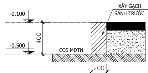
MÓNG GẠCH MG TL: 1/25
